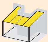
Pulldach mit Balkonausschnitt
